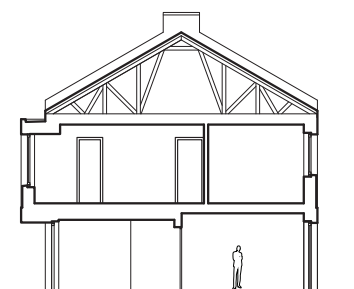
Řez domem
