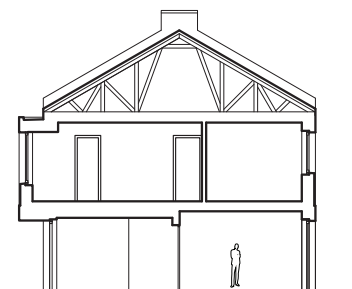
Řez domem
