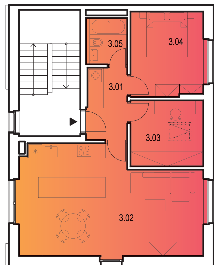
Půdorys 3.NP
