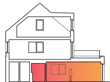
Řez, umístění jednotky v domě
